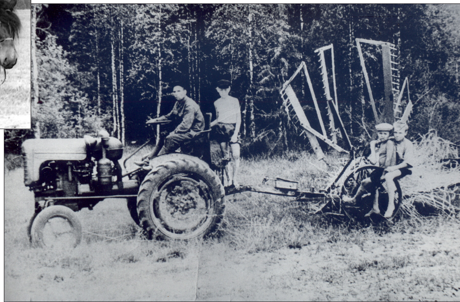
В страду помогла жатка-самосброска, агрегатируемая с трактором Т-16.
